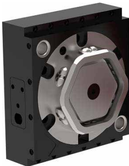
RQC Serie Roboterseite • Gewichtsbelastung: 90-550 Kg • 19 elektrische Kontakte und 6 Luftanschlüsse
