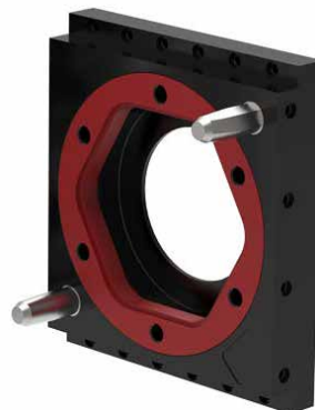
RTP Serie Werkzeugseite • Gewichtsbelastung: 90-550 Kg • 19 elektrische Kontakte und 6 Luftanschlüsse
