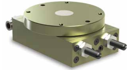
RR Serie Mittlere/schwere Betriebsart Schwenkeinheit • Hub: 0°-180° • Gewichtsbelastung: 3.6-91 Kg
