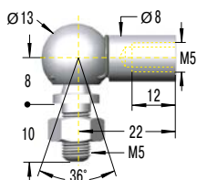
C5-VA Winkelgelenk
