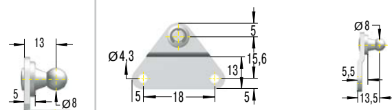
OG5-V4A Seitenbeslag
