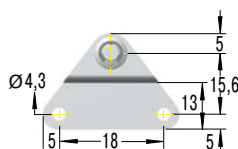
OA5-V4A Seitenbeslag
