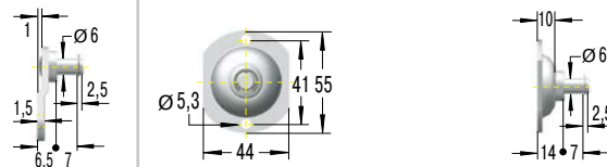
PA5-V4A Rundbeslag
