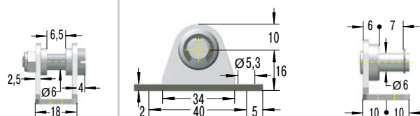
NA5-V4A Winkelbeslag
