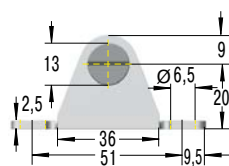
MA5-V4A Lagerschuh
