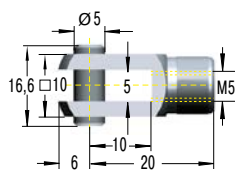
D5-VA Gabelkopf
