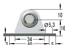
NG5-V4A Winkelbeslag
