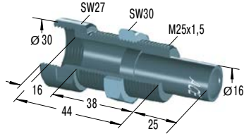
BV25 Bolzenvorlagerung
