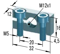
MB12 Klemmflansch
